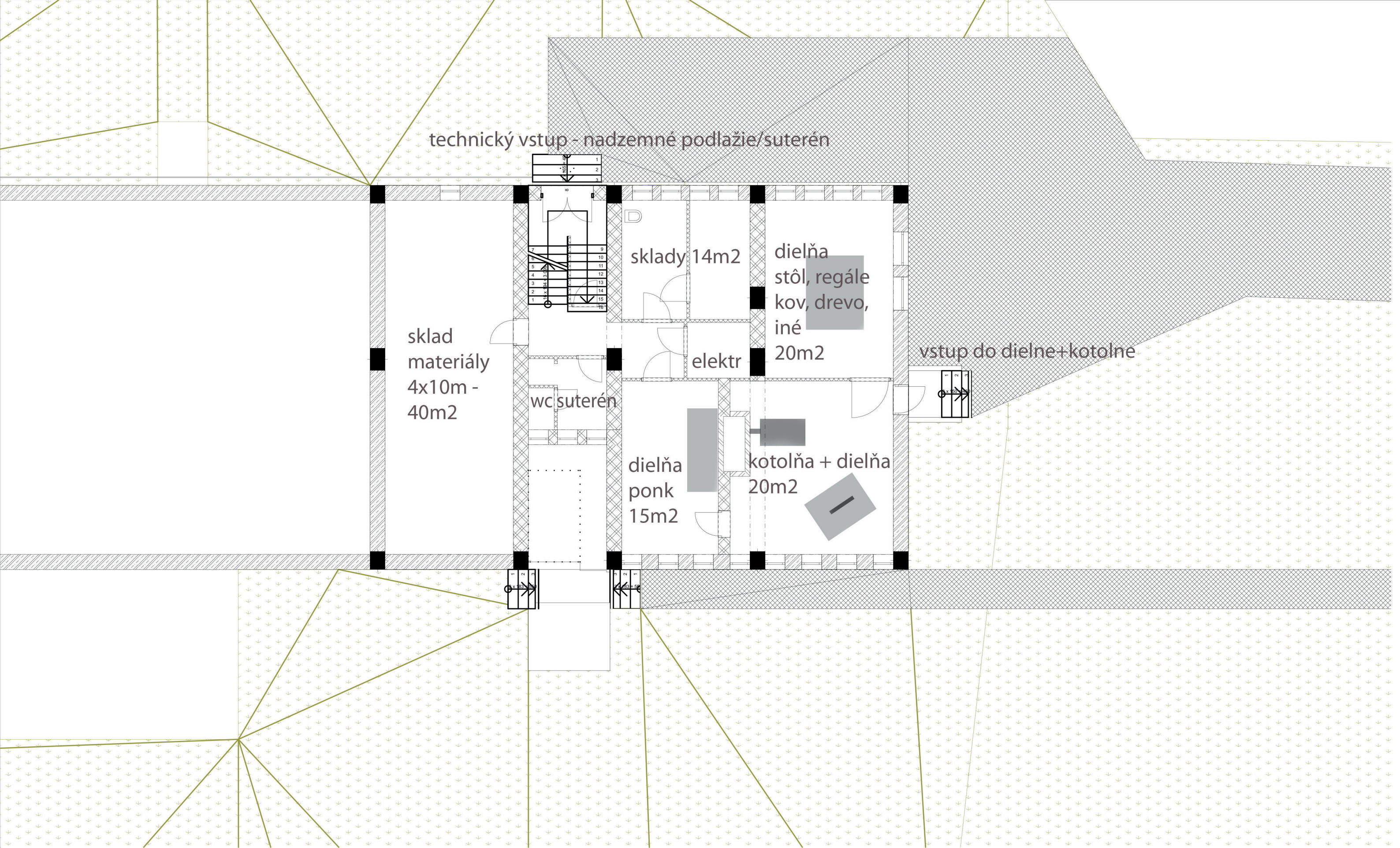
pôdorys 1. PP m 1:100
